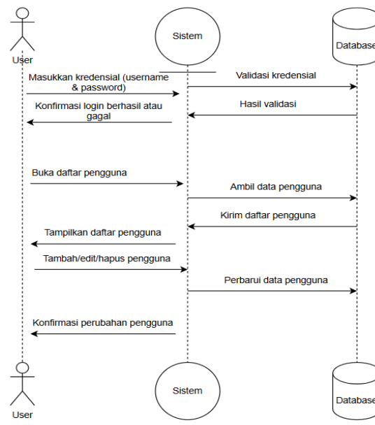
Gambar 9. Sequence Diagram Mengelola Akun Pengguna
