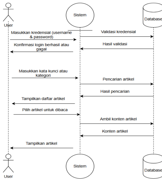
Gambar 8. Sequence Diagram Mencari Artikel Sumber: Hasil Penelitian, 2024
