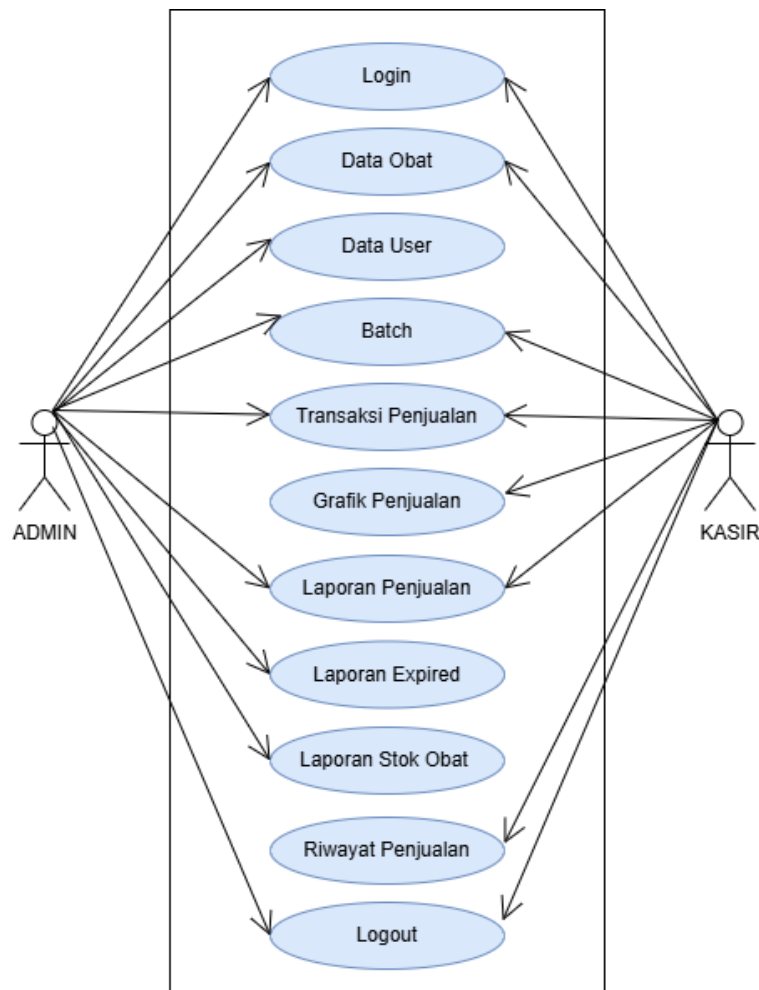
Gambar 2. Use Case Diagram Sistem Informasi Penjualan Apotek
