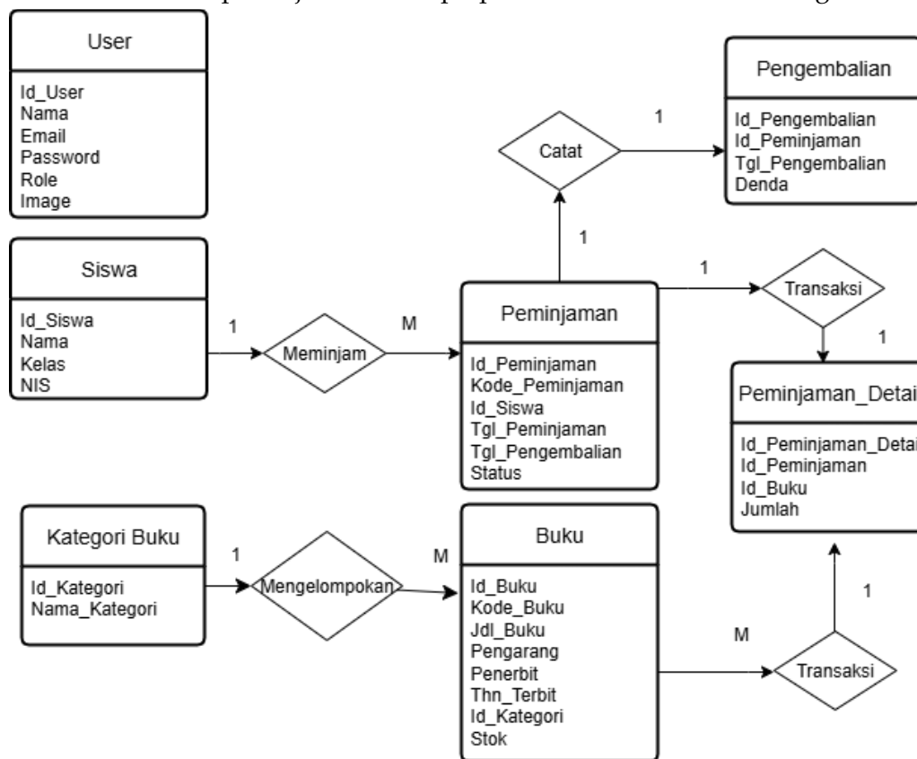
Gambar 4. ERD (Entity Row Diagram)
